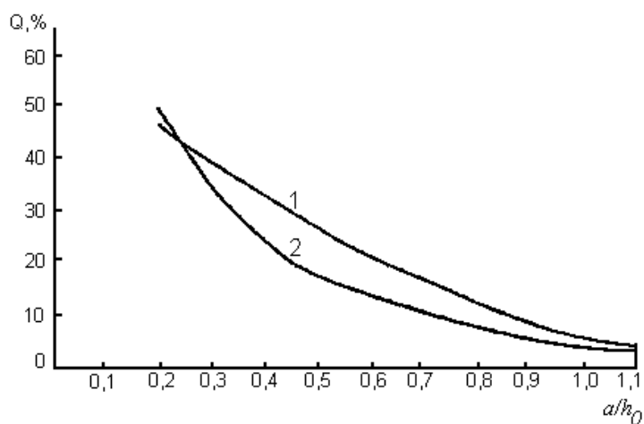
Рис.П3.3. Зависимость доли перелившейся через обвалование жидкости
