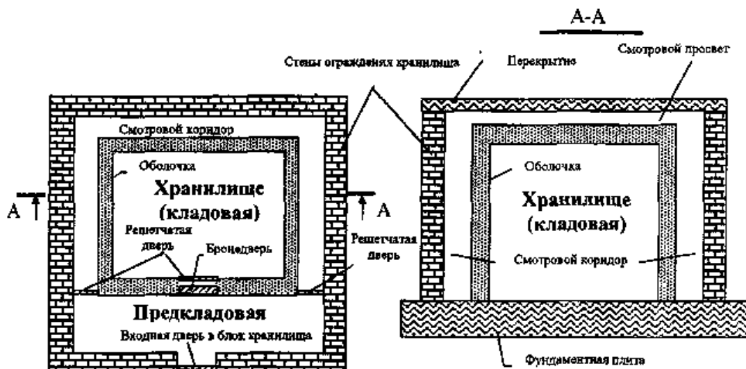
Рисунок П8.1 - Схематичное устройство хранилища ценностей
